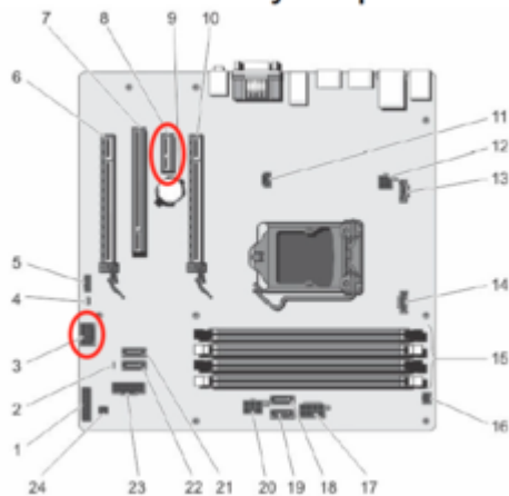
Anschlüsse auf der Systemplatine
