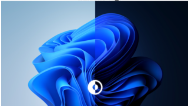
Windows 11_1
